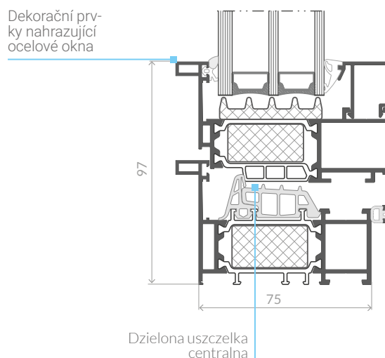
Řez oken typu INDUSTRIAL
